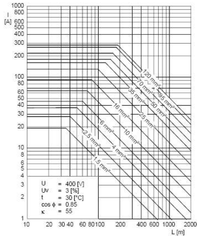
Diagramm 1: Direkt- und Anlasstrafo-Einschaltung
